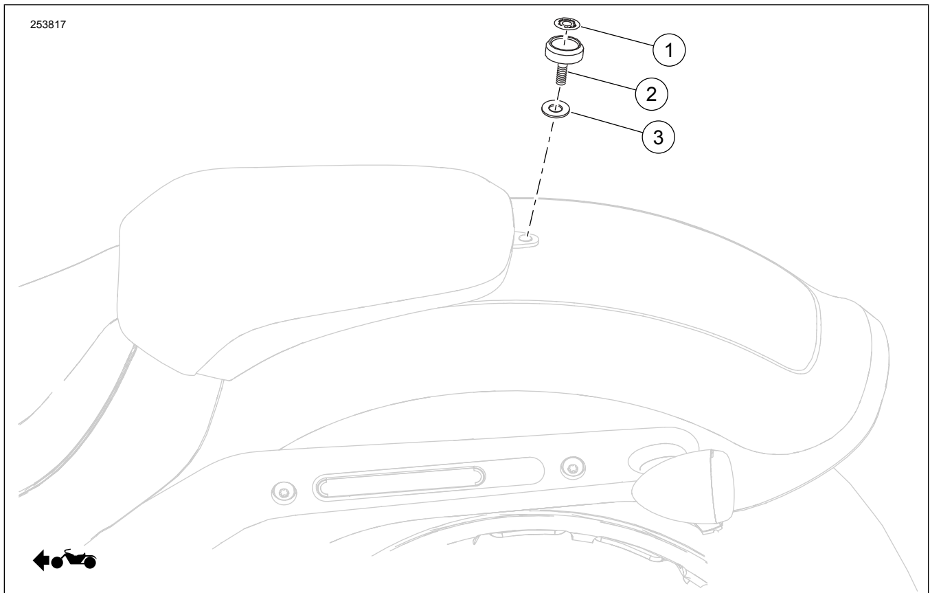
Rajah 1. Kandungan Kit: Komponen Sandaran Penunggang
