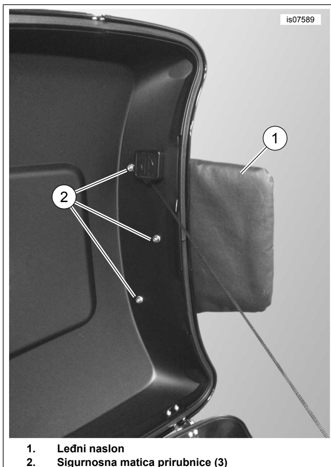
Slika 3. Postavljanje leđnog naslona na poklopcu King Tour-Pak
