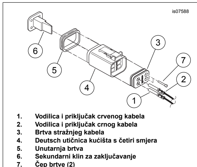
Slika 2. Umetnite priključke u Deutsch utičnicu kućišta
