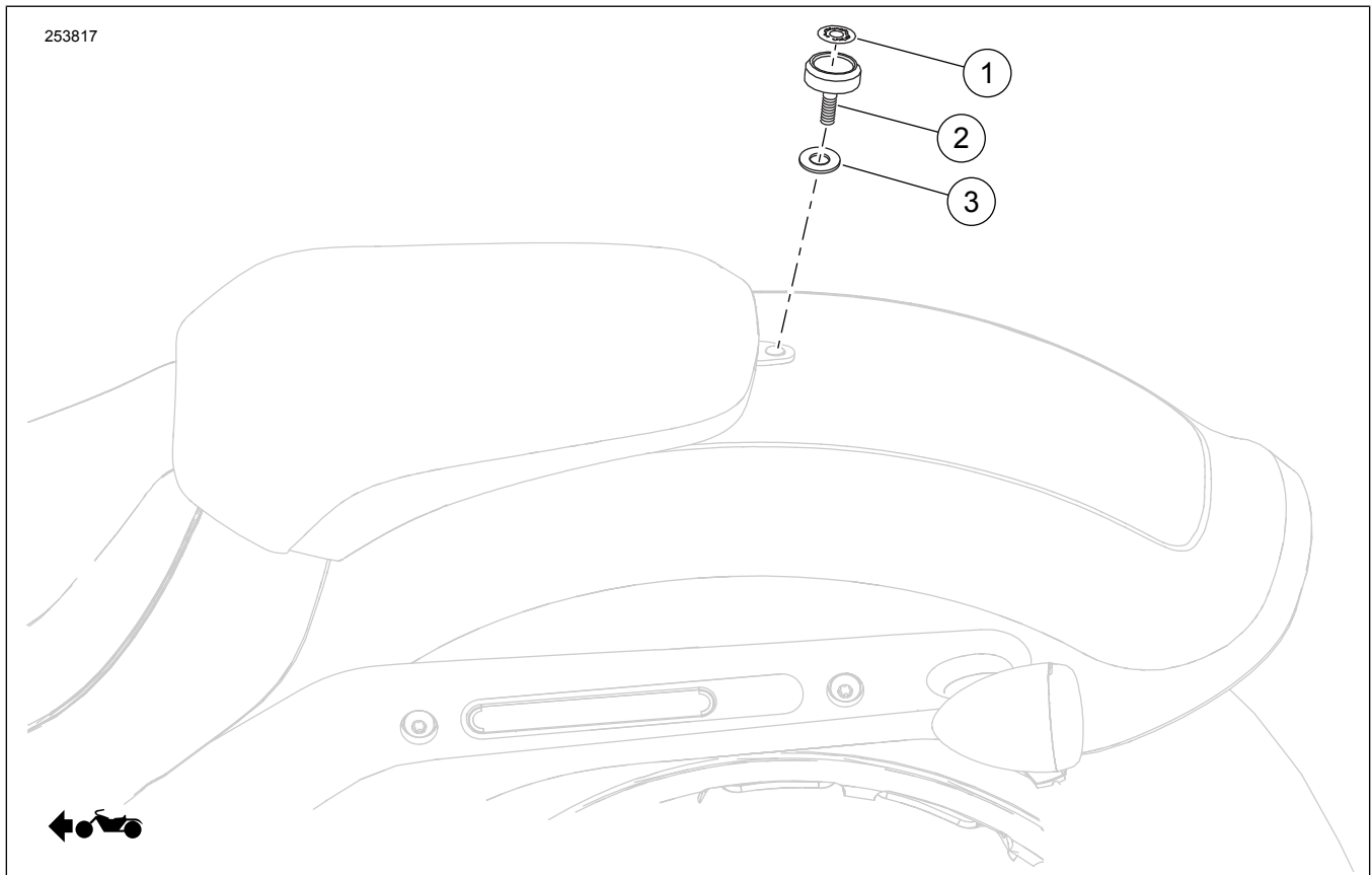
Slika 1. Sadržaj kompleta: Komponente leđnog naslona vozača
