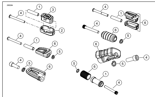
Εικόνα 1. Κιτ πείρου λεβιέ ταχυτήτων
