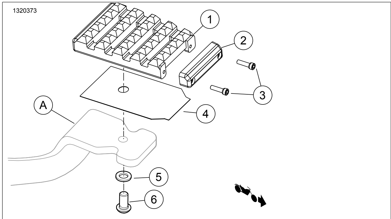
Attēls 1 Komplekta saturs: Bremžu pedāļu uzliku sastāvdaļas
