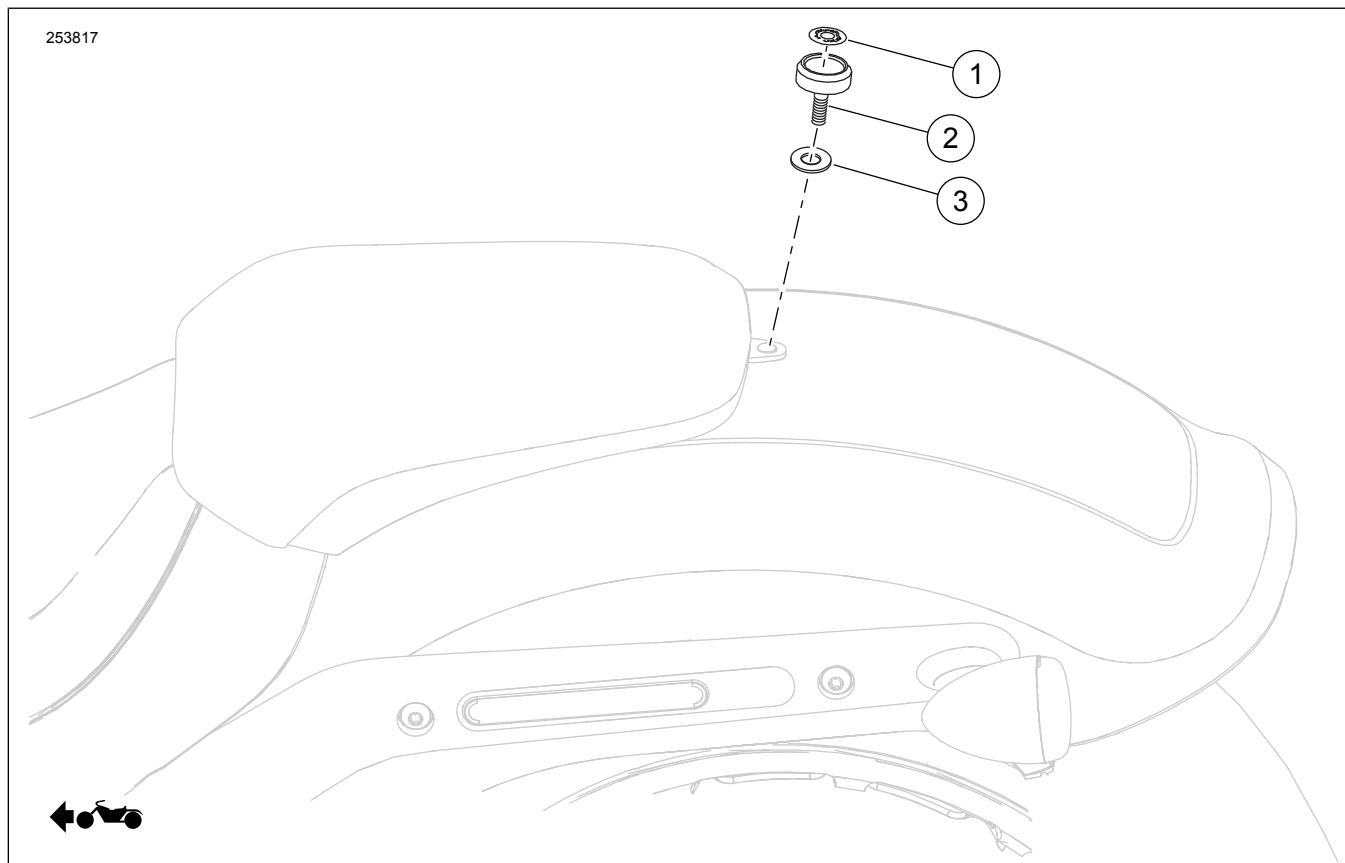
Ábra 1. A készlet tartalma: Motorvezető háttámlájának alkatrészei
