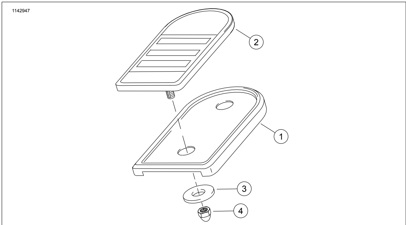
Малюнок 1. Вміст комплекту: Комплект хромових накладок гальмівних педалей – великі компоненти
