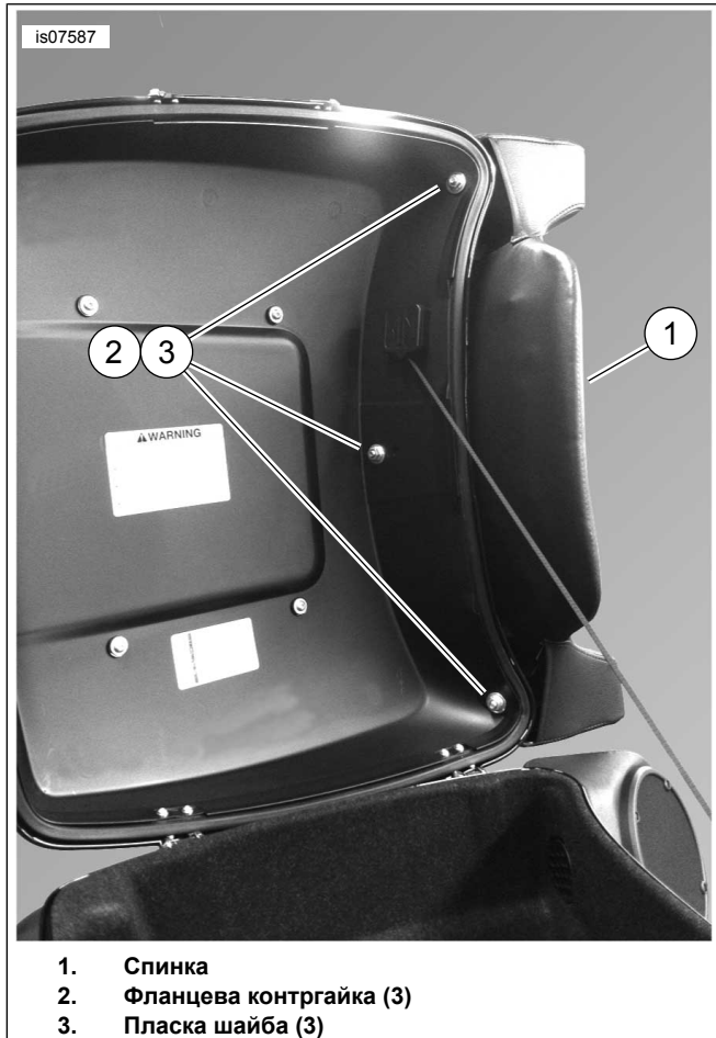
Малюнок 1. Змонтована спинка на кришці King Tour-Pak
