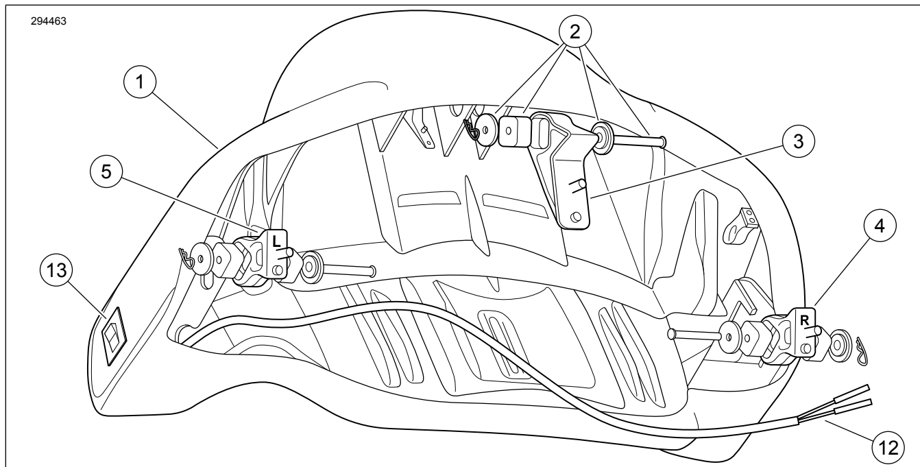
Малюнок 4. Запчастини, що обслуговуються, комплект спинки King Tour-Pak 52300312, 52300314, 52300316, 52300317, 52300334, 52300574
