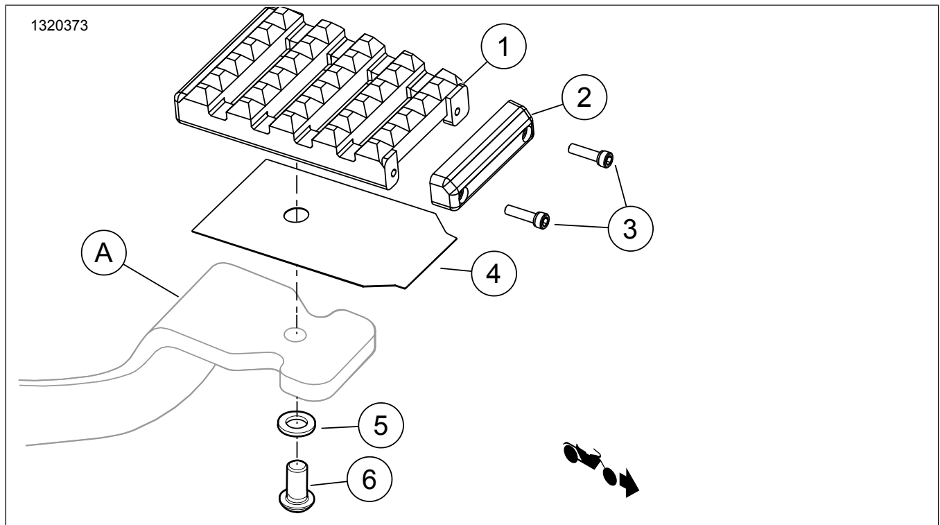
Figur 1. Settets innhold: Komponenter for bremsepedalpute
