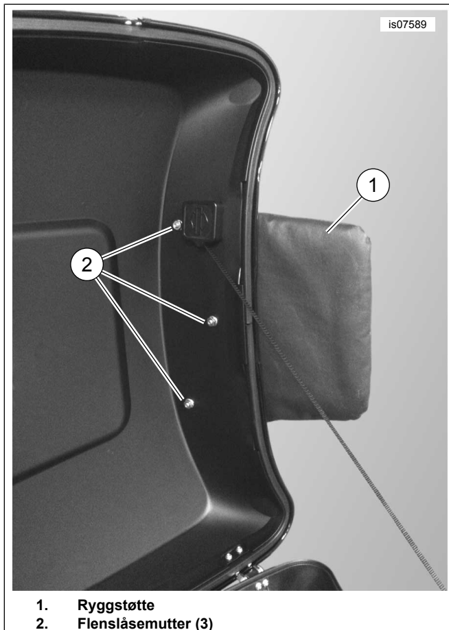
Figur 3. Montert bakhviler på Chopped Tour-Pak-lokk
