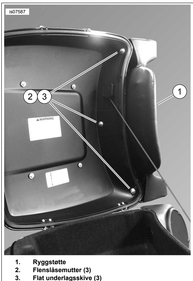
Figur 1. Montert bakhviler på King Tour-Pak-lokket
