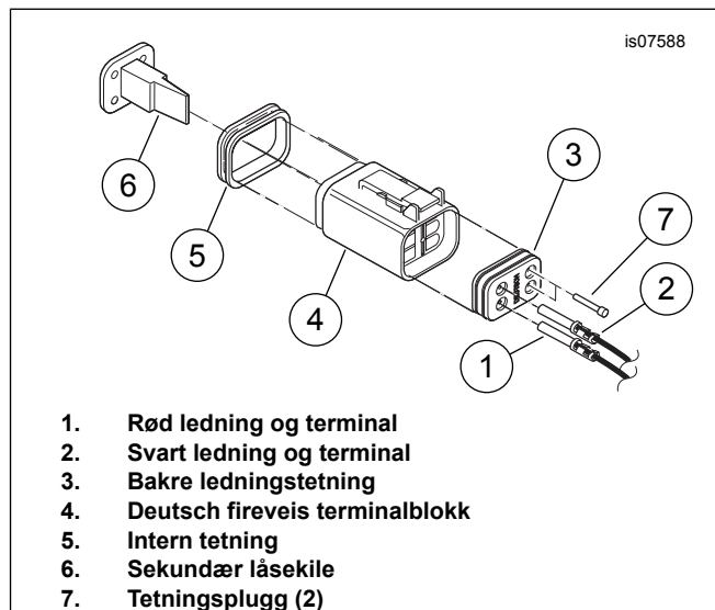
Figur 2. Sett terminaler inn i Deutsch-terminalblokk
