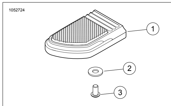
Figur 2. Servicedeler: STOR – bremsepedalpute
