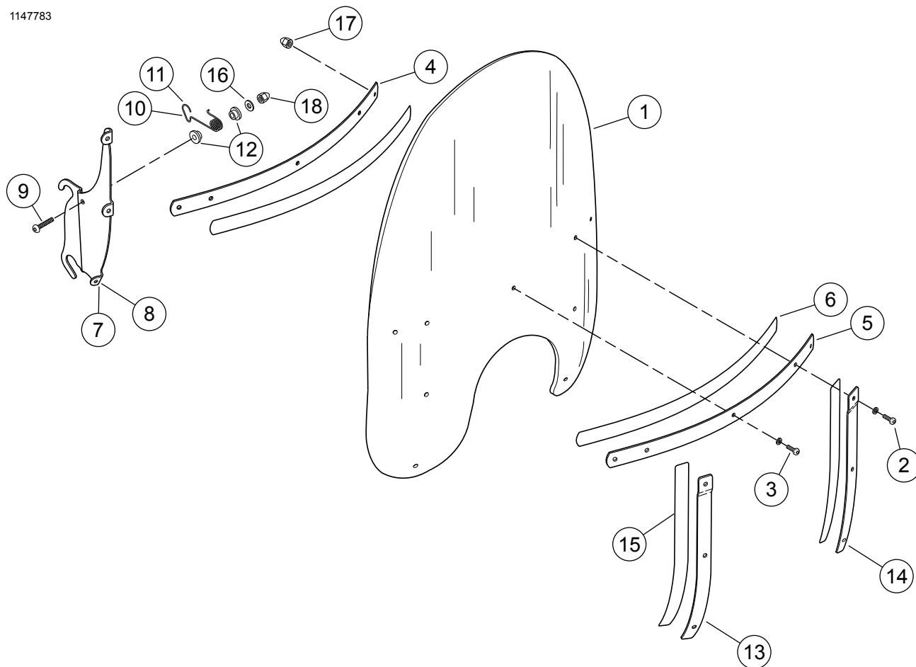
Figur 1. Servicedeler: Vindskjermenhet
