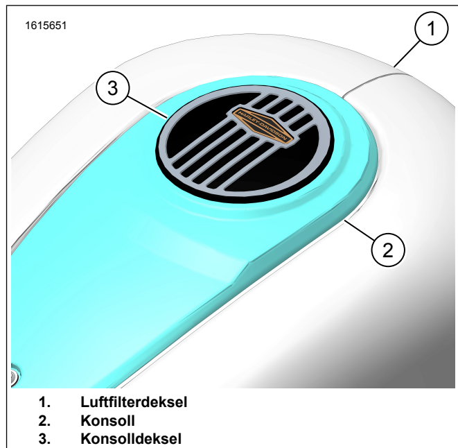
Figur 2. Konsollpynt montert
