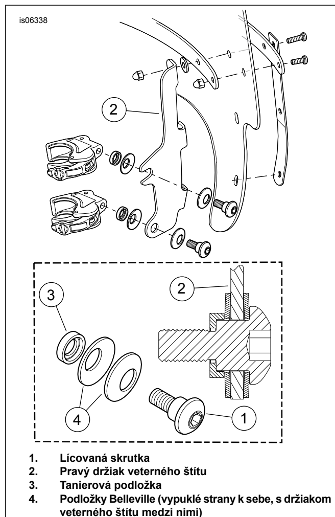
Obrázok 1. Montážne príchytiky veterného štítu (zobrazená pravá strana)
