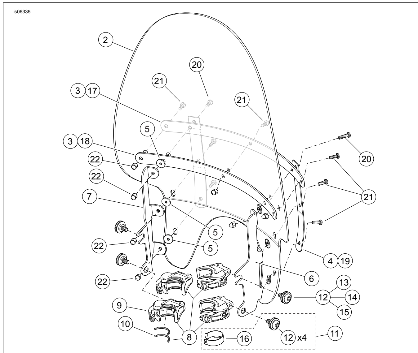
Obrázok 2. Servisné diely, rýchlosnímateľný veterný štít XL1200X
