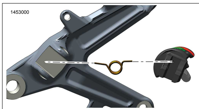
Obrázok 5. Orientácia vratnej pružiny – pravá strana
