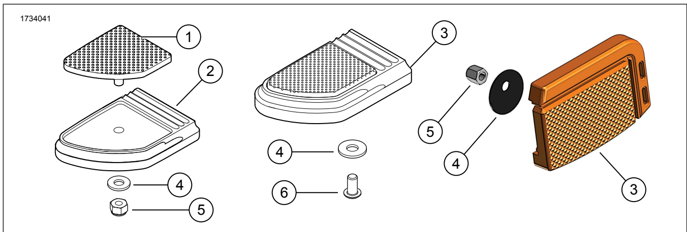
Obrázok 1. Obsah súpravy: Súprava vložky brzdového pedála
