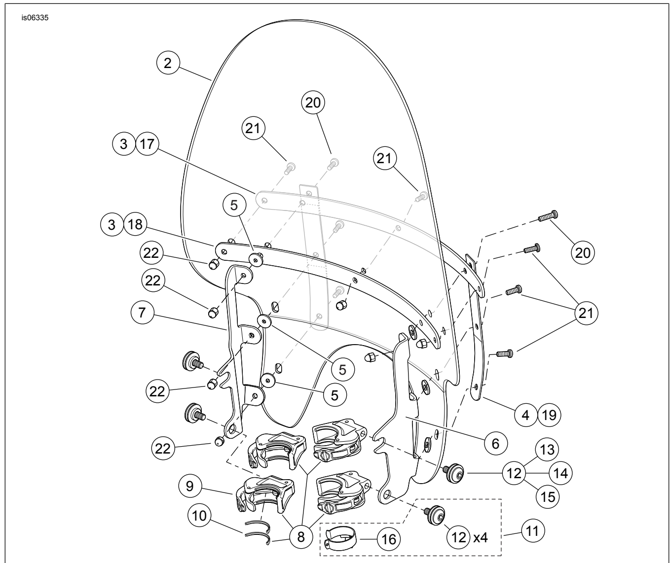
Slika 2. Servisni deli, vetrobran s hitro sprostitevijo XL1200X
