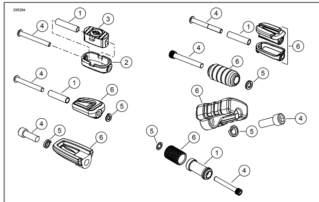
Рисунок 1. Комплект педали рычага переключения передач
