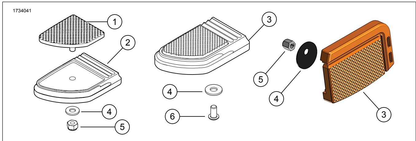
Рисунок 1. Содержимое комплекта Комплект накладок педали тормоза
