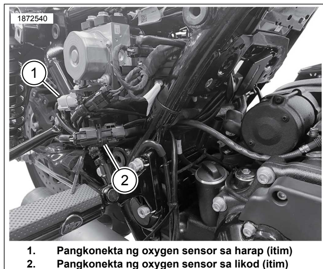
Figure 4. Mga Koneksyon ng Pangunahing Harness ng ATM
