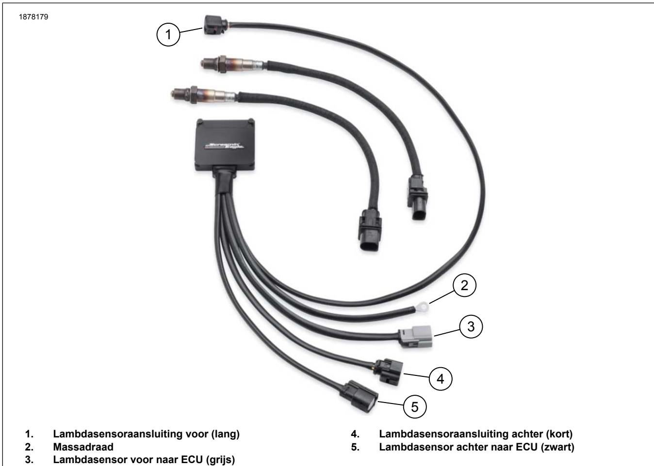
Afbeelding 53. Beschreven kabelboomaansluitingen
