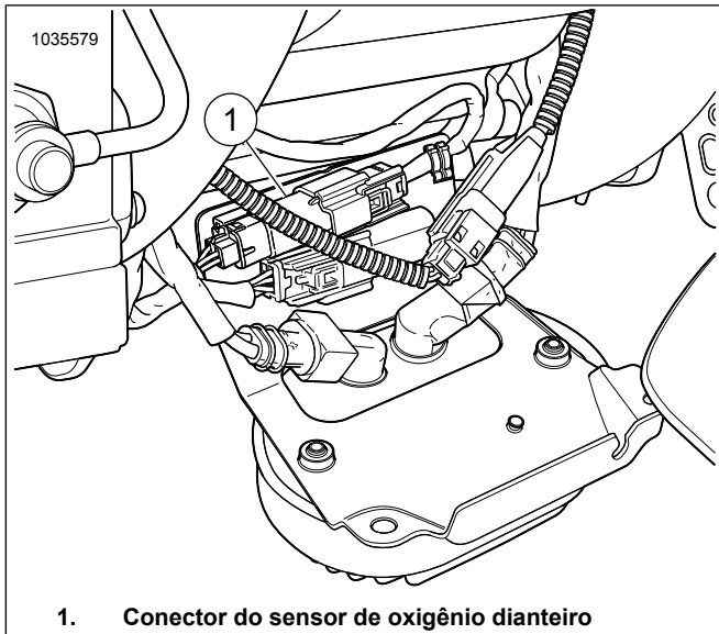
1. Conector do sensor de oxigênio dianteiro Figura 32. Localização do sensor de oxigênio dianteiro
