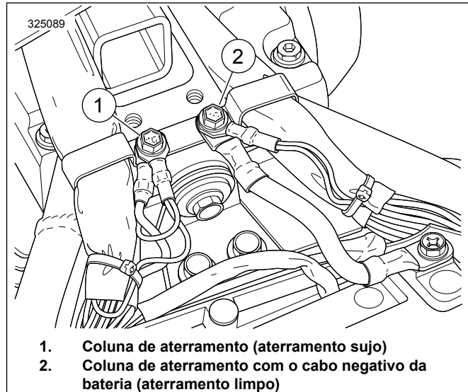
Figura 34. Localizações da coluna de aterramento na caixa de bateria
