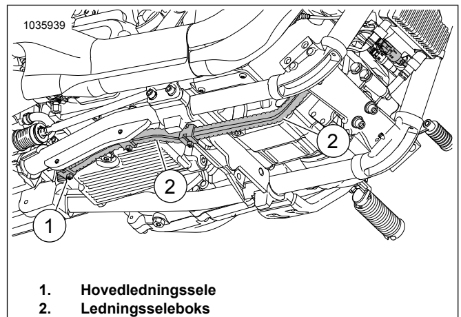
Figur 44. Ledningsseleboks
