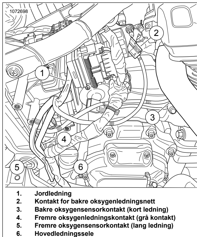
Figur 24. Trekking av ATM-ledningsselle
