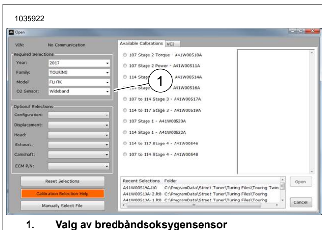
Figur 26. Valg av bredbåndsoksygensensor
