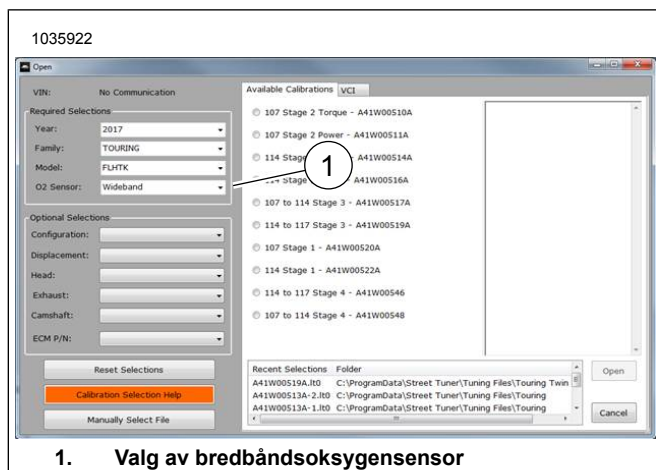
Figur 17. Valg av brendbåndsoksygensensor
