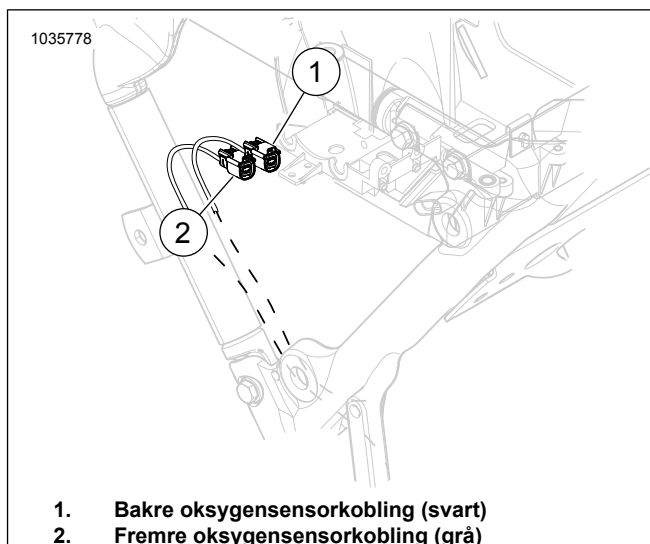
Figur 1. Plassering av fremre og bakre oksygensensor
