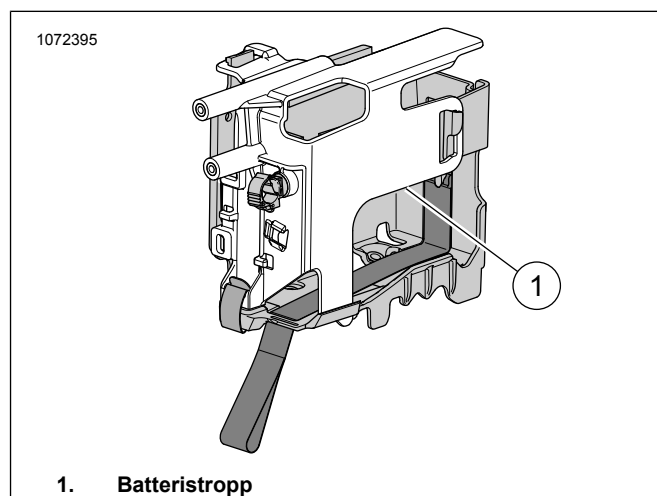
Figur 19. Plassering av batteristroppen
