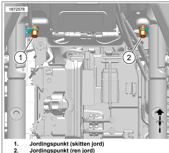
Figur 7. Plassering av jordingspunkter for batteriet
