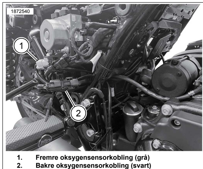
Figur 4. ATM-hovedledningsselekontakter
