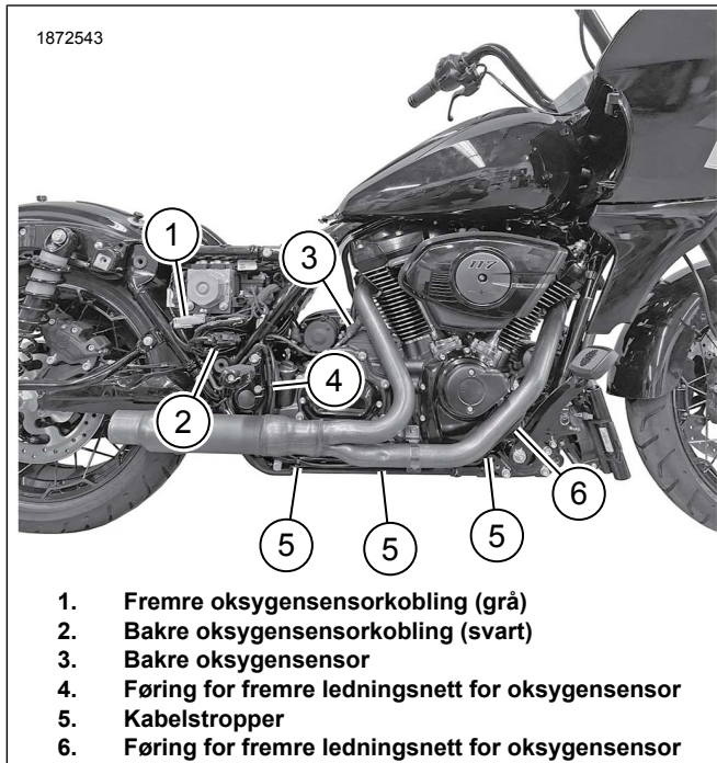
Figur 8. Trekking av ATM-sensorledningssele
