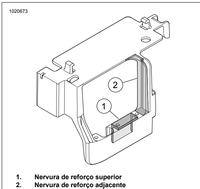
Figura 28. Áreas destacadas para serem cortadas
