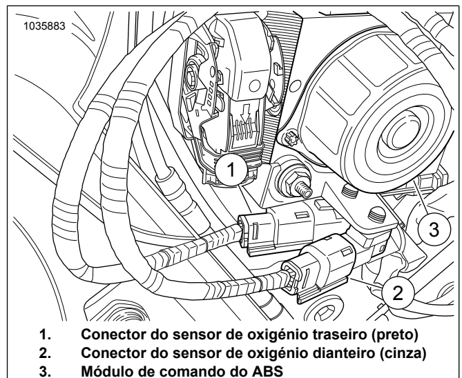
Figura 13. Conectores da cablagem principal do ATM
