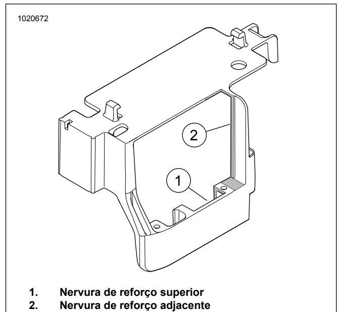
Figura 30. Parte de trás da armação cortada
