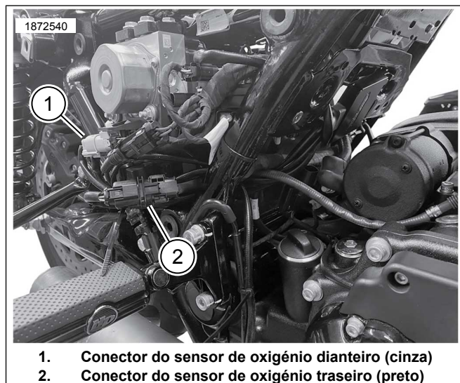
Figura 4. Conectores da cablagem principal do ATM
