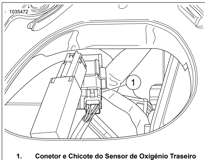
1. Conector e Chicote do Sensor de Oxigénio Traseiro
