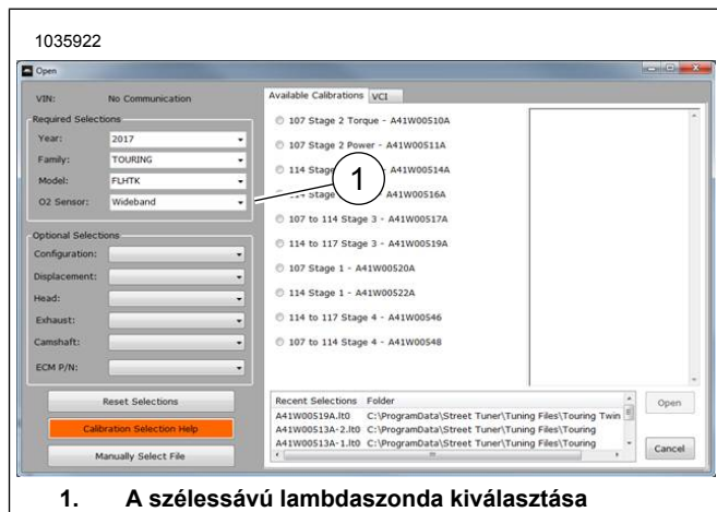
Ábra 9. A széles sávú lambdaszonda kiválasztása
