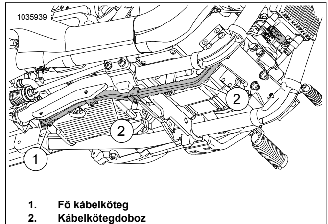
Ábra 44. Kábelkötegdoboz
