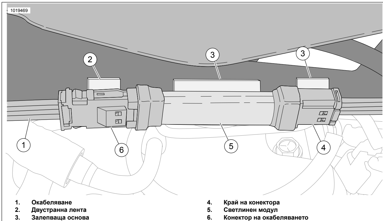
Фигура 1. Светлинен модул, конектори и двустранна лента
