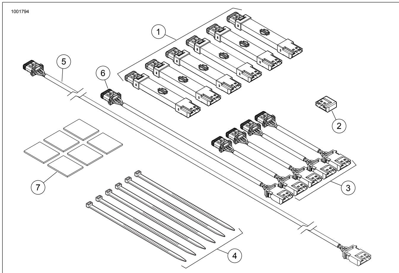
Фигура 2. Части за обслужване, комплекти светлинни модули Spectra Glo
