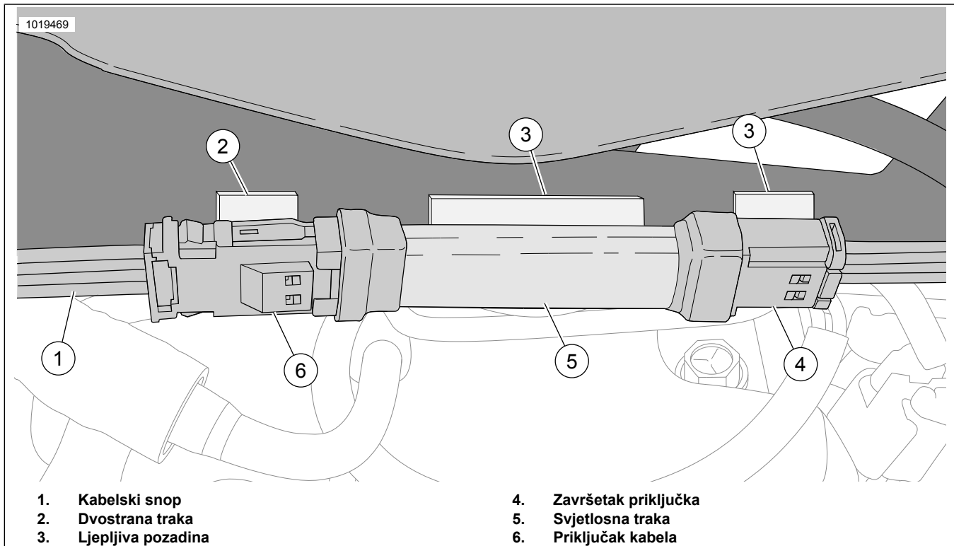
Slika 1. Svjetlosna jedinica, konektori i dvostrano ljepljiva traka
