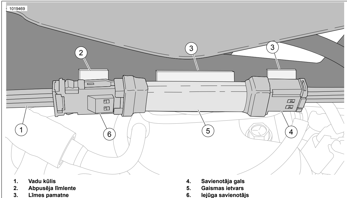
Attēls 1 Gaismas kapsula, savienotāji un divpusēja lente
