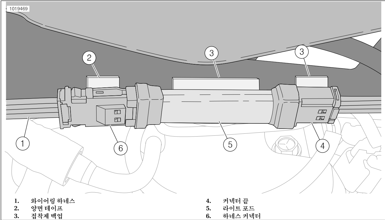
그림 1. 라이트 포드, 커넥터 및 양면 테이프
