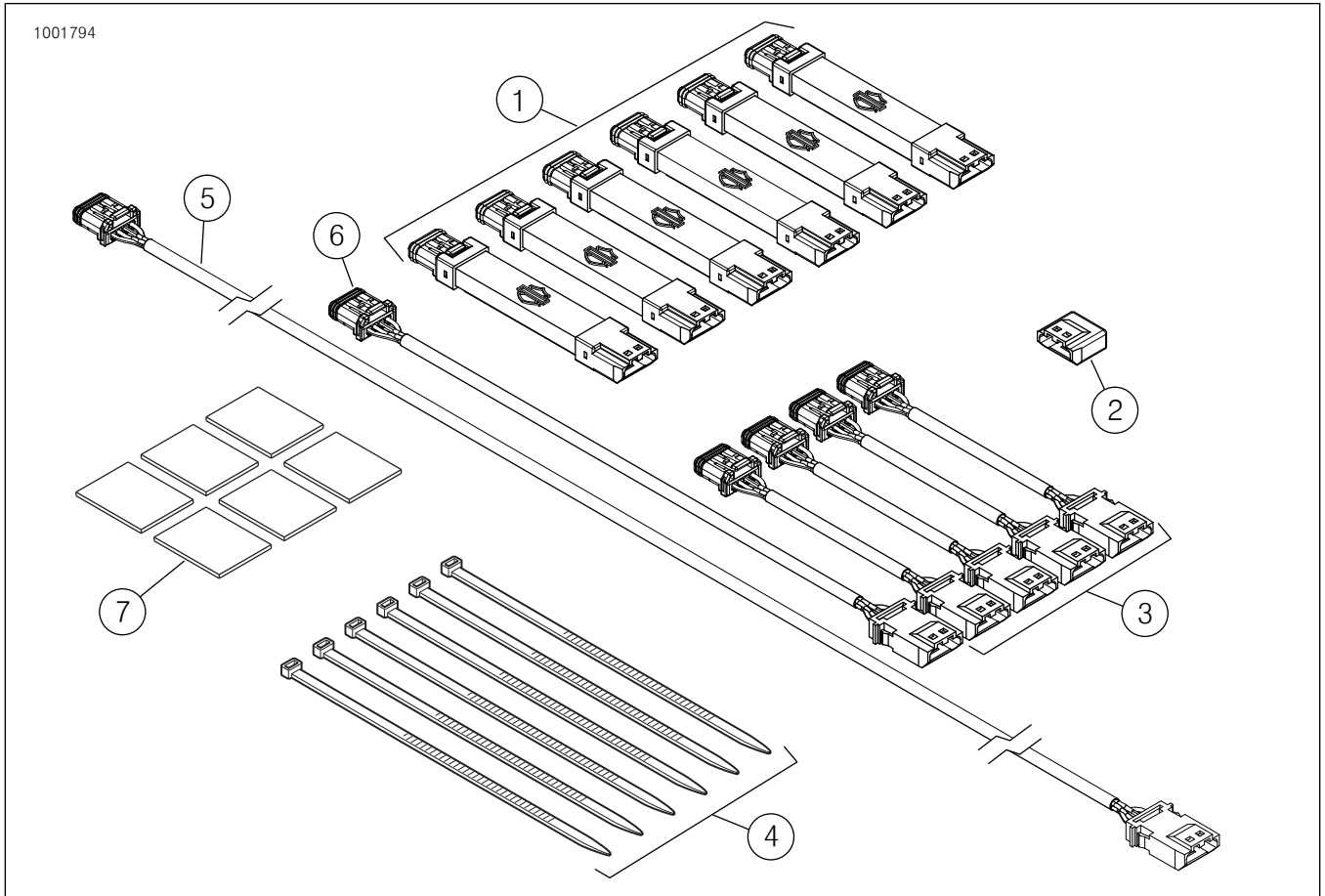
그림 2. 정비 부품, Spectra Glo 라이트 포트 키트
