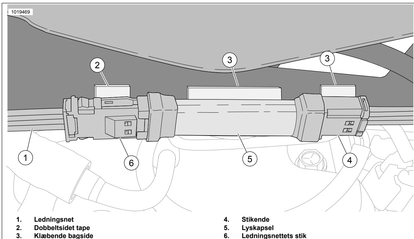
Figur 1. Lygtereflektor, stik og dobbeltklæbende tape
