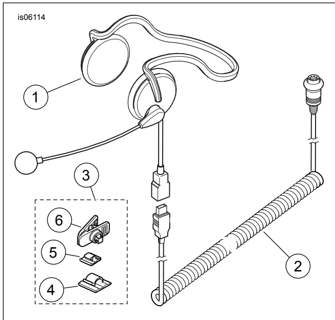
Gambar 2. Komponen Servis, Headset Musik dan Komunikasi Helm Half Face
