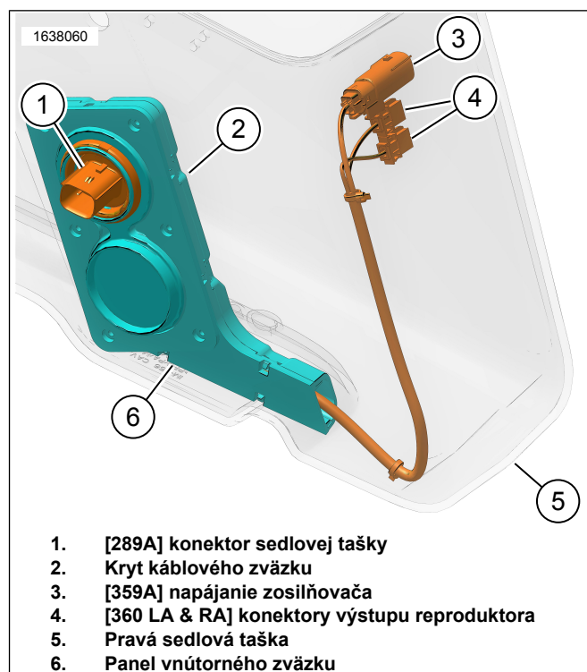
Obrázok 8. Vnútorný káblový zväzok 69202871
