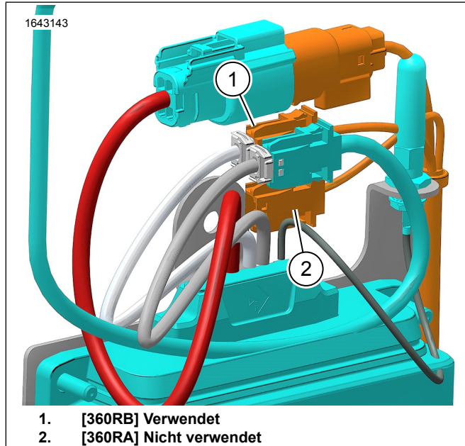
Abbildung 6. Lautsprecher [360RA] und [360RB]
