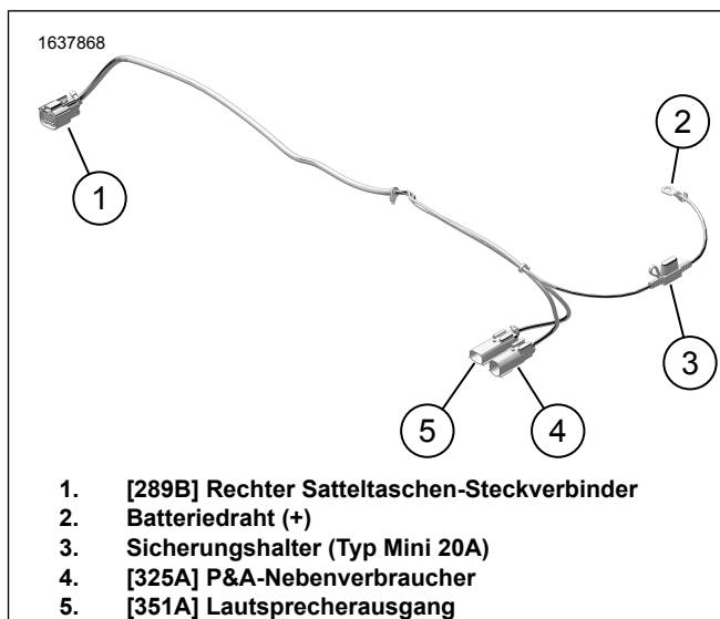
Abbildung 15. Externer Kabelbaum 69202870
