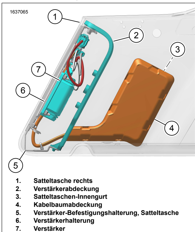
Abbildung 13. Satteltaschenkabelbaum mit Verstärker
