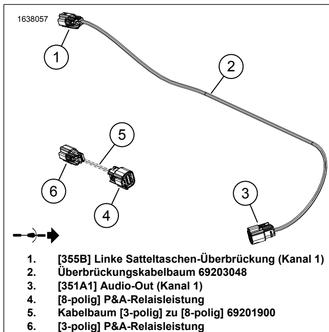
Abbildung 16. Überbrückungskabelbaum
