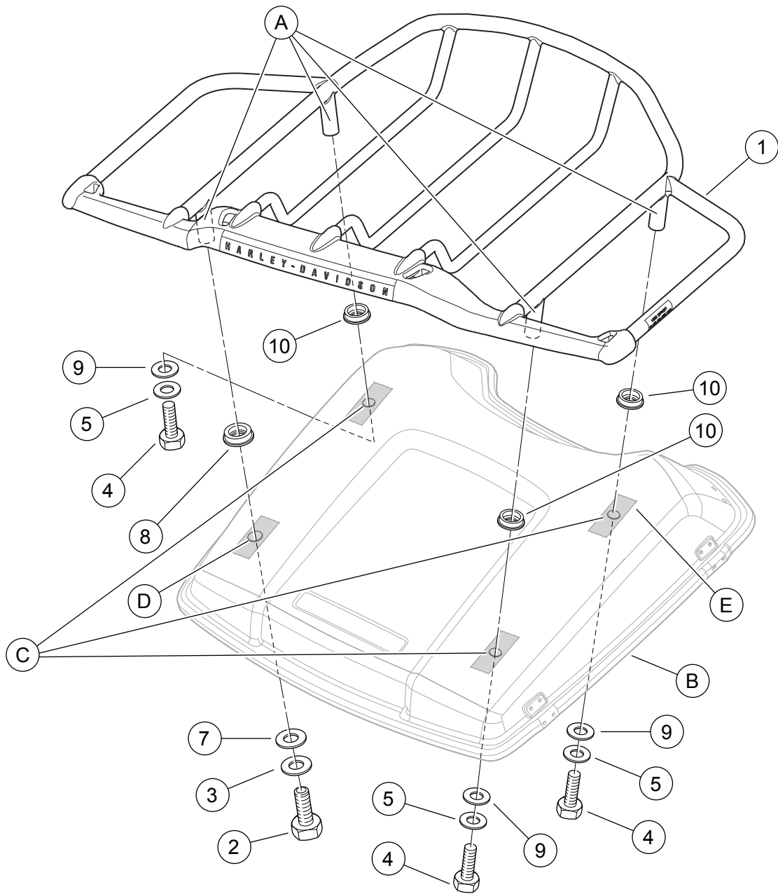
Attēls 1 Apkopes daļas, Air Wing Tour-Pak vāka statīvs
