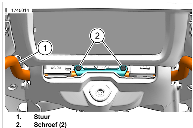
Afbeelding 2. Stuurschroef
