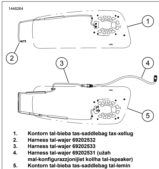
Figura 2. Konfigurazzjoni u Routing tal-Harness tal-Wajer
