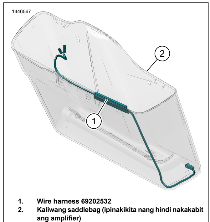
Figure 8. Pagruruta ng Harness ng Kaliwang Saddlebag
