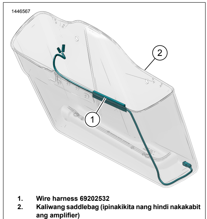
Figure 4. Pagruruta ng Harness ng Kaliwang Saddlebag
