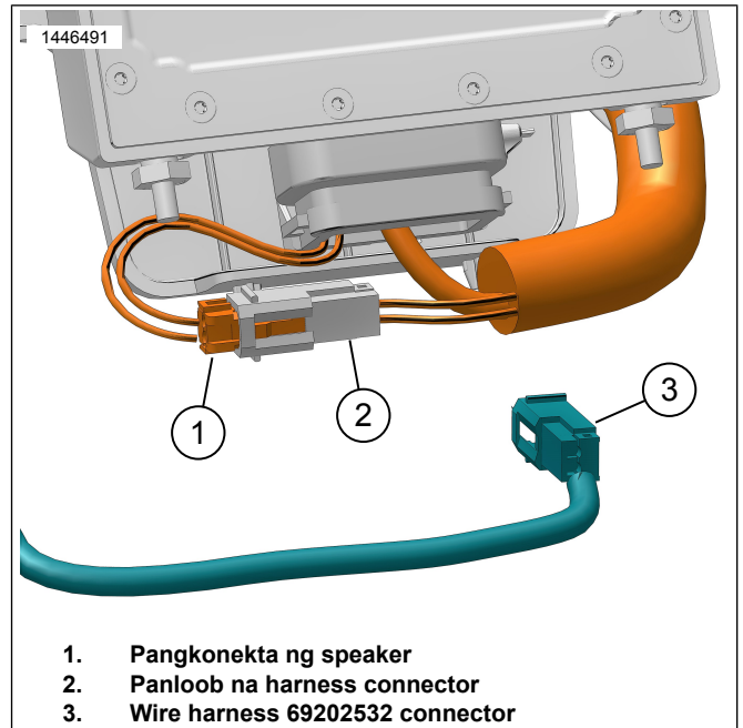
Figure 3. Koneksyon ng Speaker ng Kaliwang Saddlebag
