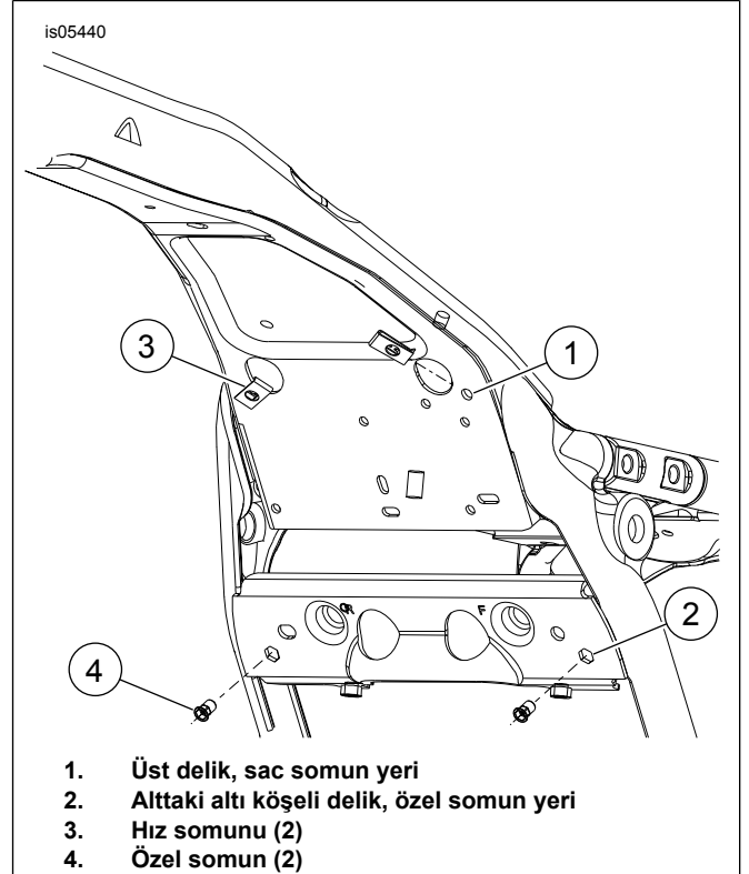
Şekil 1. Bağlayıcıların Yeri
