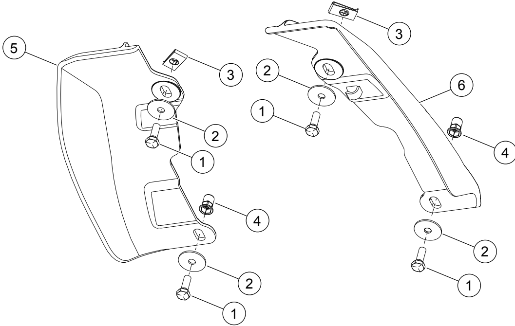
Şekil 3. Servis Parçaları: Orta Şasi Hava Deflektörleri
