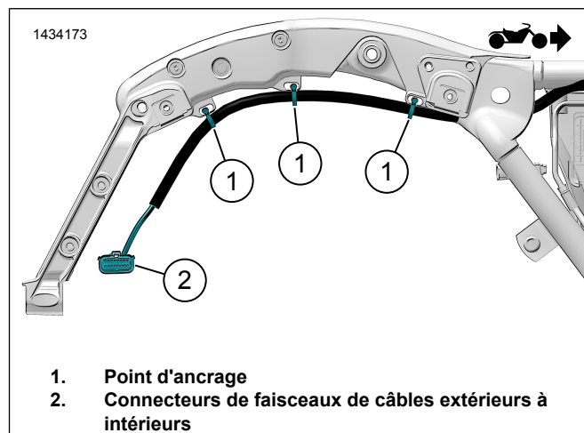
Figure 17. Acheminement du faisceau de fils extérieur (typique)
