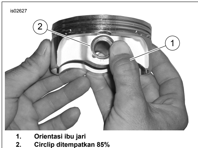
Gambar 4. Pemasangan Circlip
