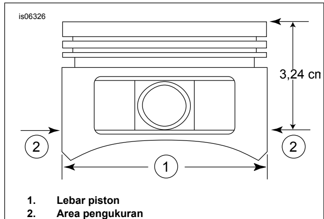
Gambar 2. Pengukuran Piston
