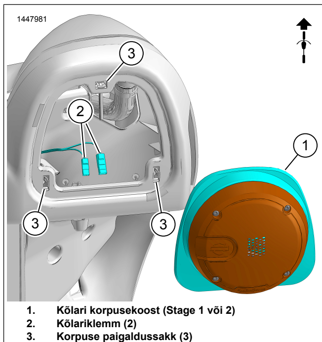
Joonis 2. Gondli alaosa kõlarite paigaldamine
