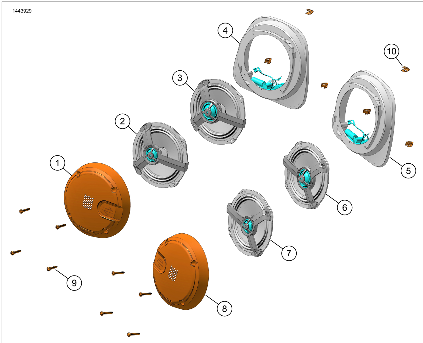
Joonis 4. Varuosad, gondli alaosa kölarid
