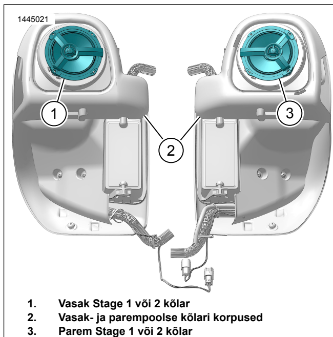
Joonis 3. Kaksikjahutusega kõlari orientatsioon
