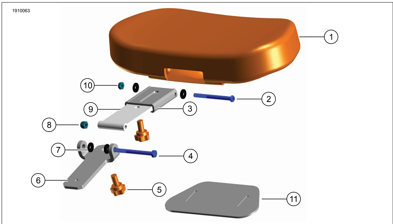
Figura 1. Conținut kit: Spătar - Pilot
