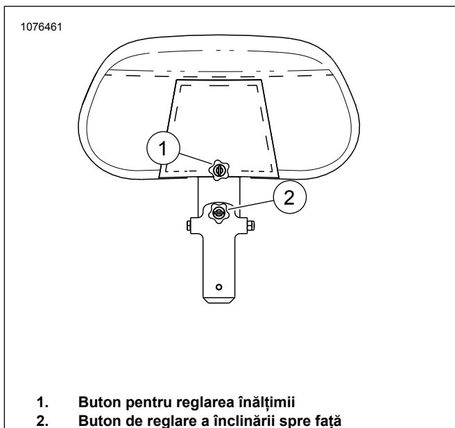
Figura 3. Butoane de reglare a spătarului pentru pilot
