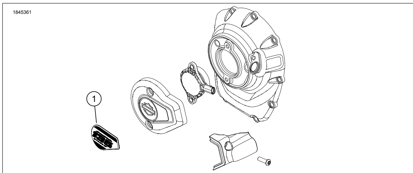
Figure 1. Contenu du kit : Médaille de carter d'allumage Screamin' Eagle
