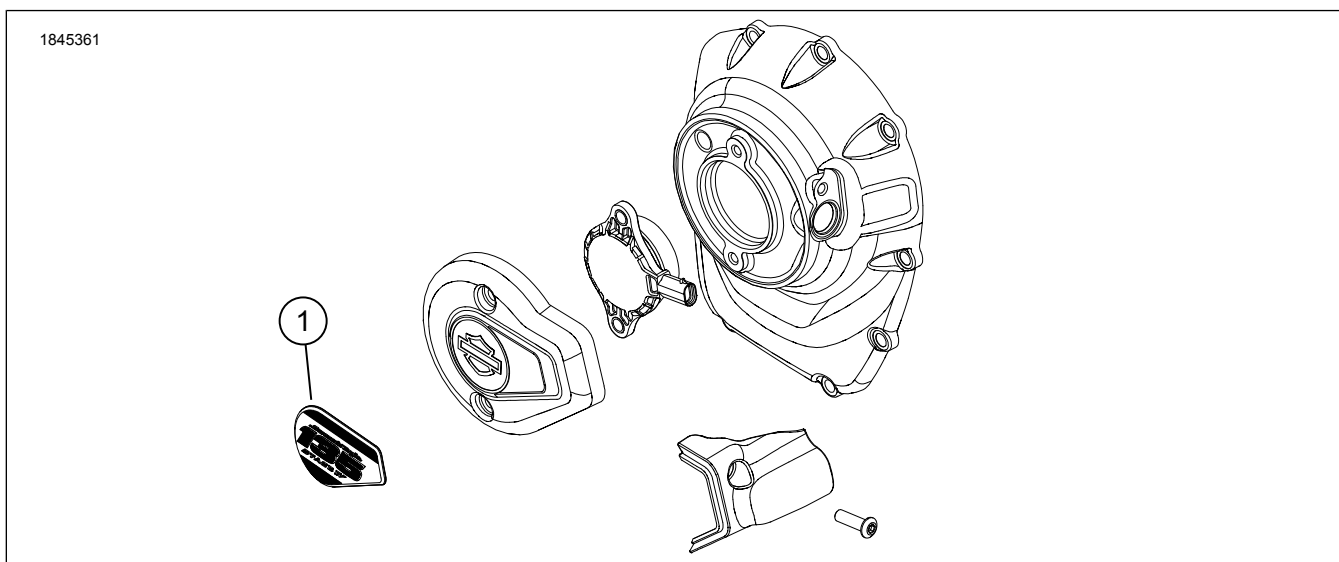
Figure 1. Contenu du kit : Médaillon de carter de distribution Screamin' Eagle
