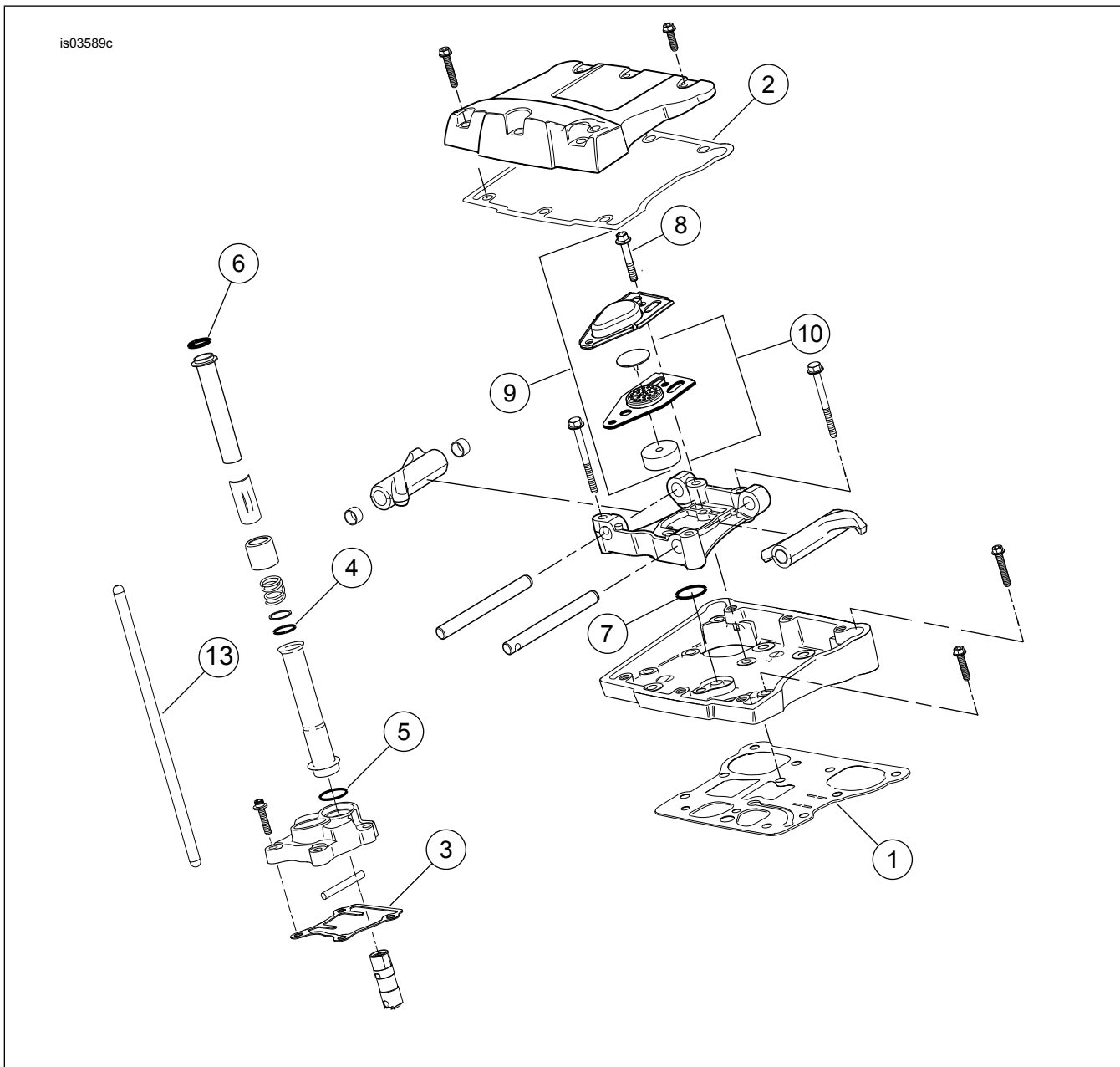
Figure 2. Mga Pamalit na Piyesa: Screamin' Eagle Pro TC 103 (96 CI hanggang 103 CI) Stage 4 Kit
