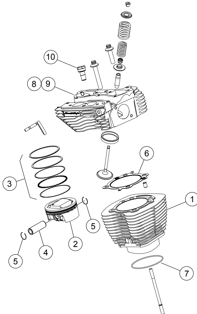
Ábra 1. Szervizelhető alkatrészek: Screamin' Eagle Pro TC 103 (96-103 CI) Stage 4. készlet
