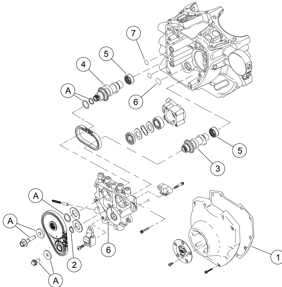
Ábra 3. Szervizelhető alkatrészek: Screamin' Eagle Pro TC 103 (96–103 CI) Stage 4. készlet
