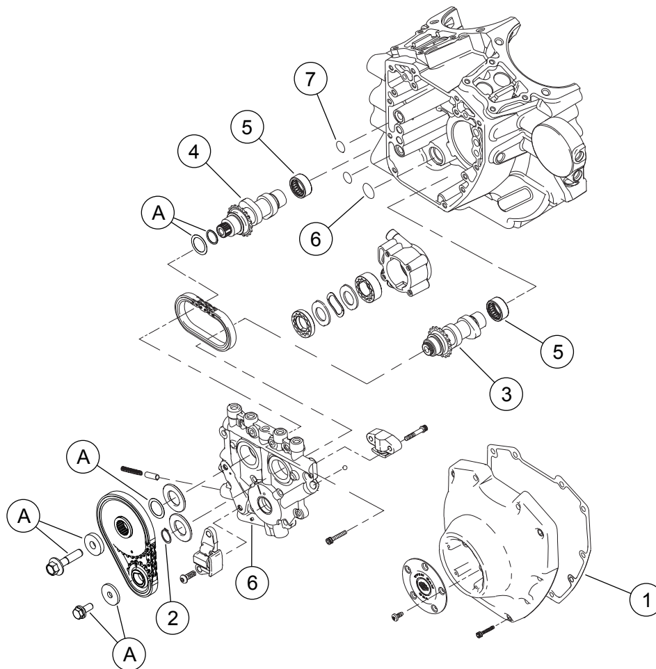
Attēls 3 Apkopes daļas: Screamin' Eagle Pro TC 103 (96 TI līdz 103 CI) 4. posma komplekts
