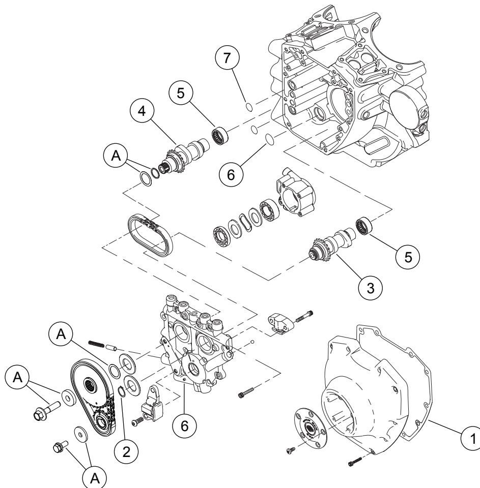
Figura 3. Componente de service: Kit Etapa 4 Screamin' Eagle Pro TC 103 (96 CI până la 103 CI)
