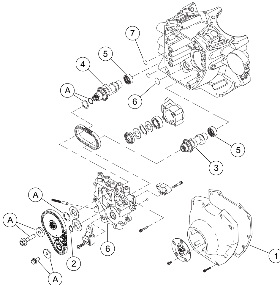
Figur 3. Reservdelar: Screamin' Eagle Pro TC 103 (96 CI till 103 CI) Steg 4-sats
