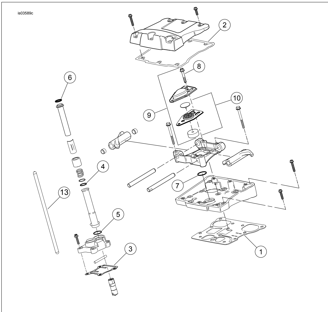
Figur 2. Reservdelar: Screamin' Eagle Pro TC 103 (96 CI till 103 CI) Steg 4-sats
