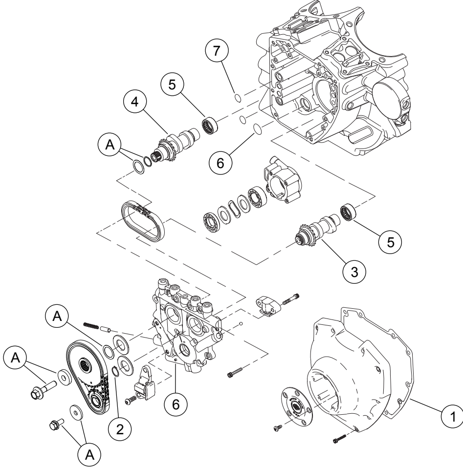
Şekil 3. Servis Parçaları: Screamin' Eagle Pro TC 103 (96 CI to 103 CI) Stage 4 Kiti
