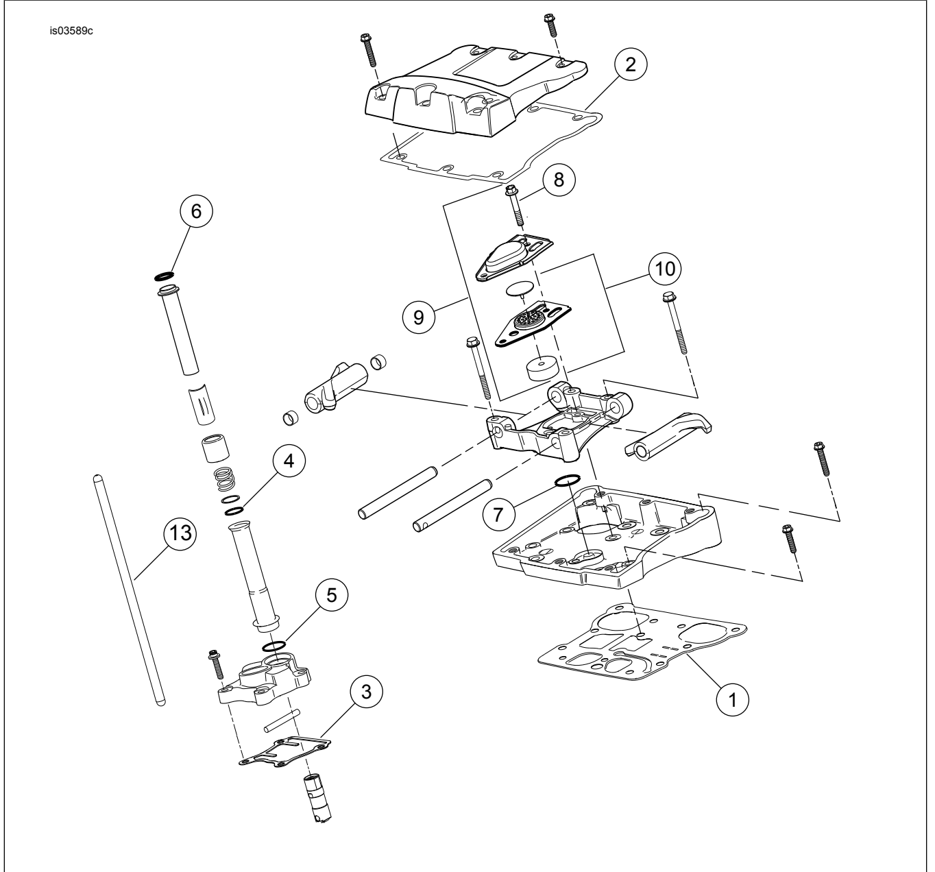
Şekil 2. Servis Parçaları: Screamin' Eagle Pro TC 103 (96 CI to 103 CI) Stage 4 Kiti
